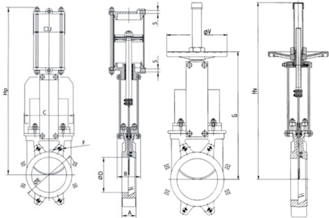
Con cilindro pneumatico / With pneumatic cylinder Avec vérin pneumatique / Mit Pneumatikzylinder
